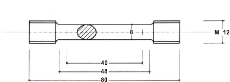
a) Probeta de tracción
