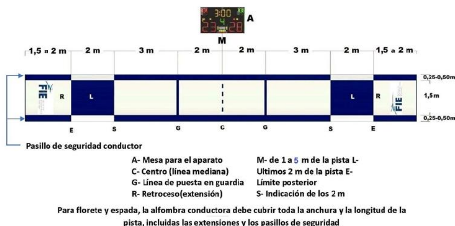
Figura 1 - PISTA PARA LAS FINALES (altura de la pista máximo 0,50 m)
